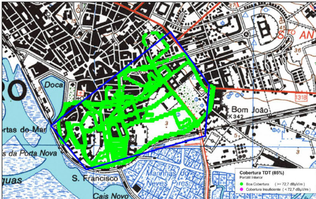
Mapa de Cobertura TDT Portátil Interior
