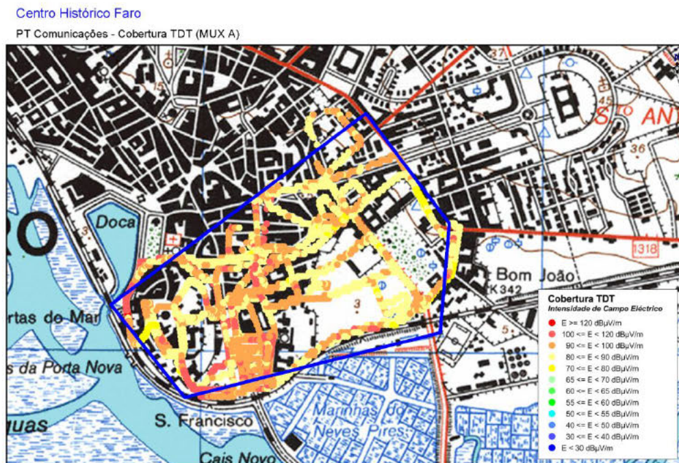
Mapa de Intensidade de Campo Elétrico
