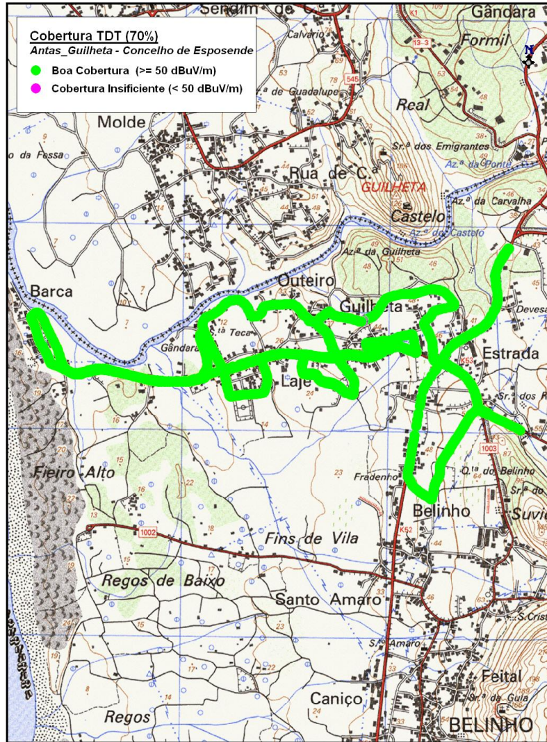
Mapa de Cobertura Fixa Exterior TDT
