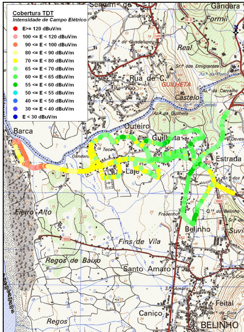
Mapa de Intensidade de Campo Elétrico
