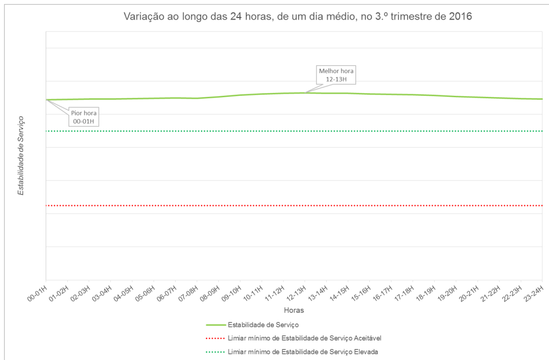
Figura 35 – Estabilidade de Serviço, nas 24 horas de um dia médio, do 3.º trimestre de 2016
