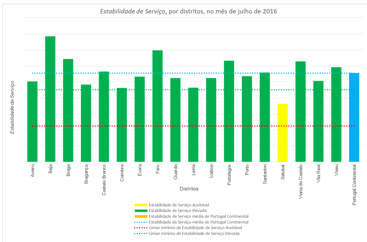
Figura 45 – Gráfico da Estabilidade de Serviço, por distritos, no mês de julho de 2016
