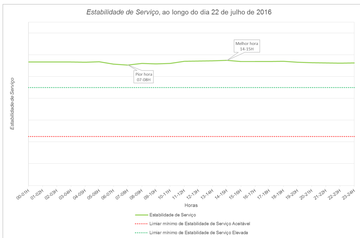
Figura 29 – Estabilidade de Serviço, ao longo do melhor dia de julho de 2016
