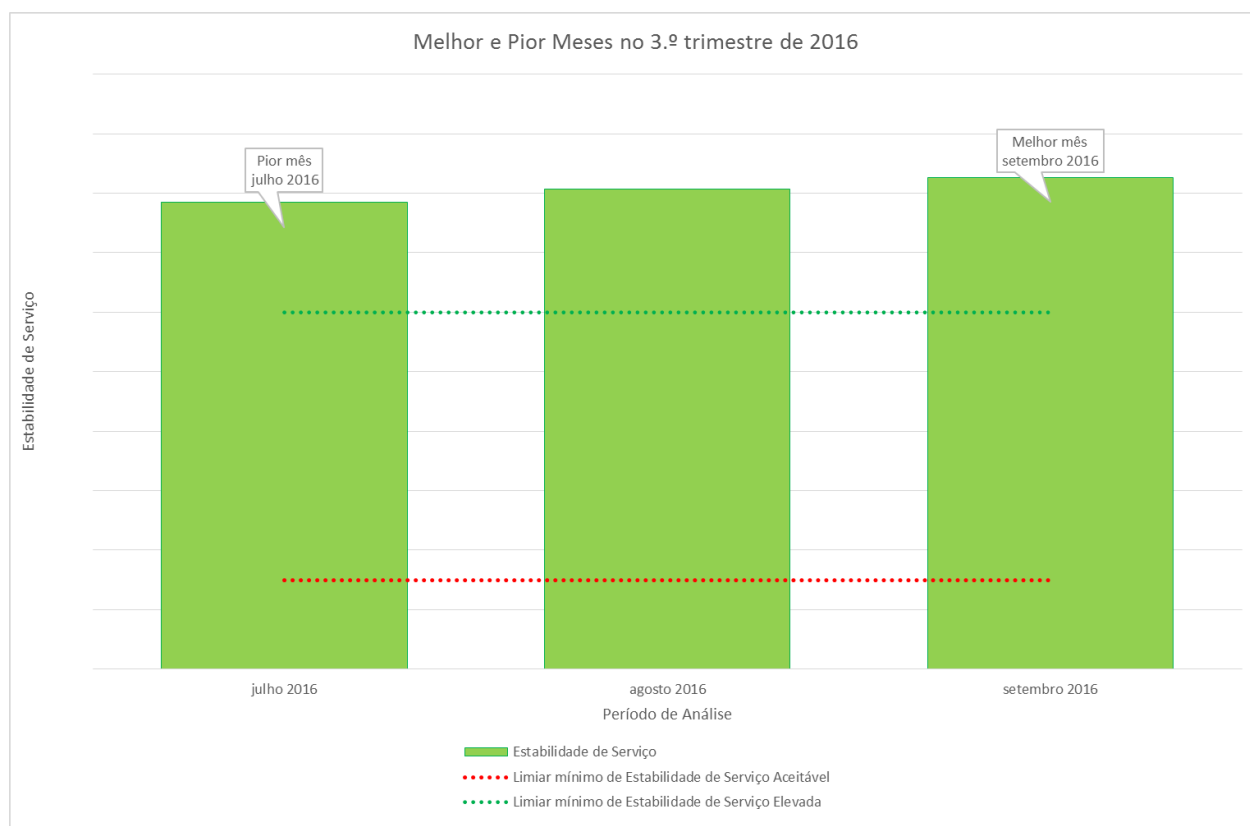
Figura 24 – Estabilidade de Serviço, em cada mês do 3.º trimestre de 2016
