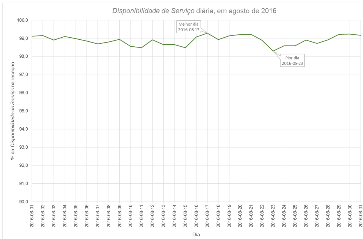
Figura 8 – Disponibilidade de Serviço em cada dia, no mês de agosto de 2016
