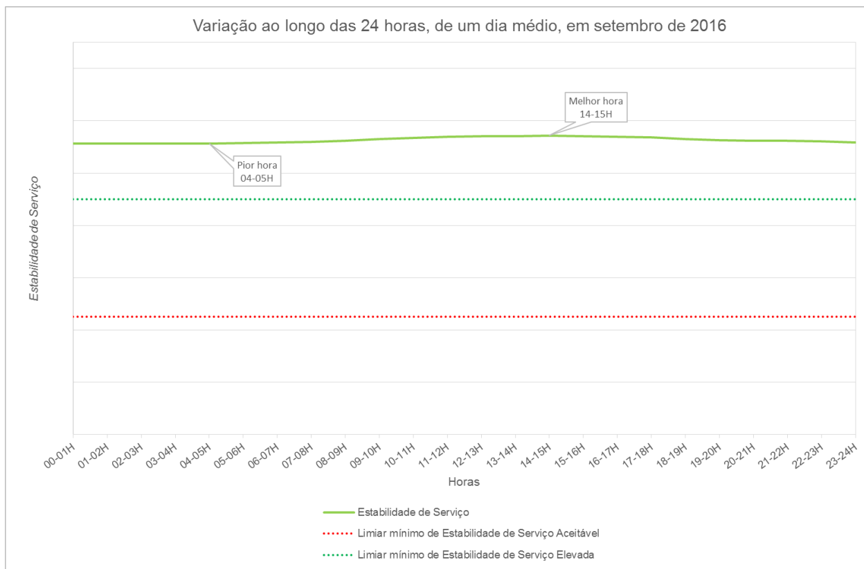
Figura 38 – Estabilidade de Serviço, nas 24 horas de um dia médio, do mês de setembro de 2016
