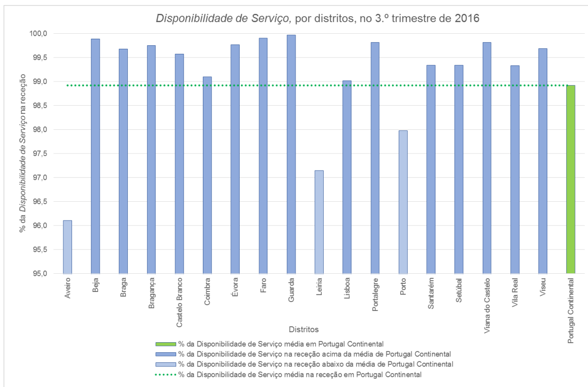
Figura 16 – Gráfico da Disponibilidade de Serviço, por distritos, no 3.º trimestre de 2016
