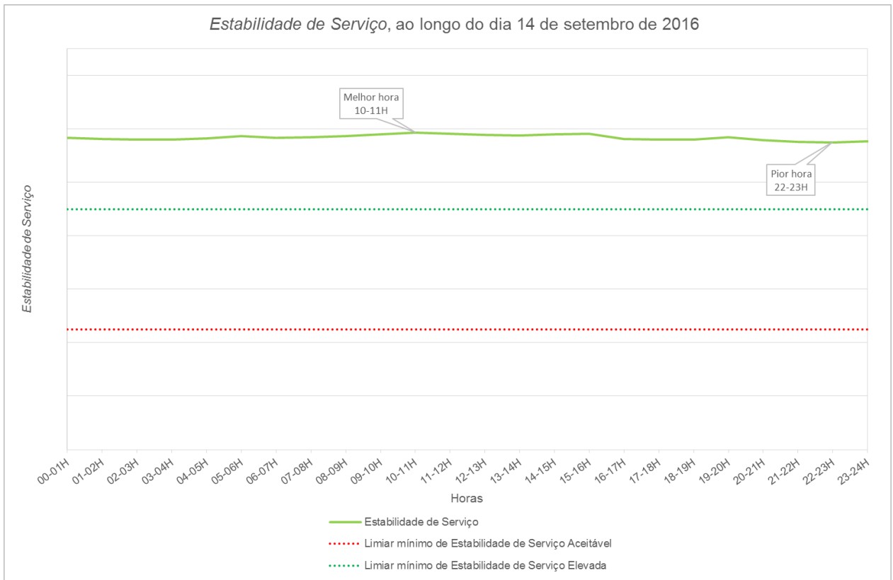
Figura 31 – Estabilidade de Serviço, ao longo do melhor dia de setembro de 2016
