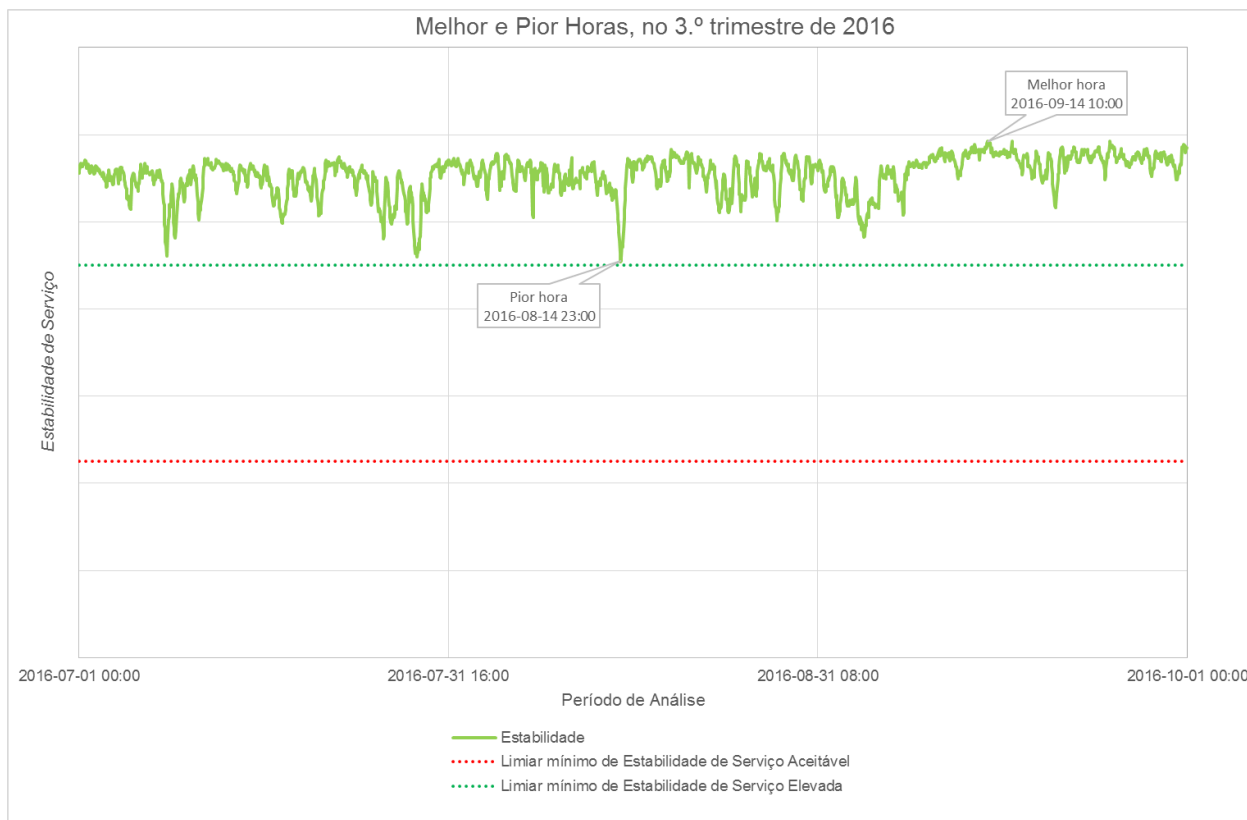
Figura 39 – Estabilidade de Serviço, hora a hora, ao longo do 3.º trimestre de 2016
