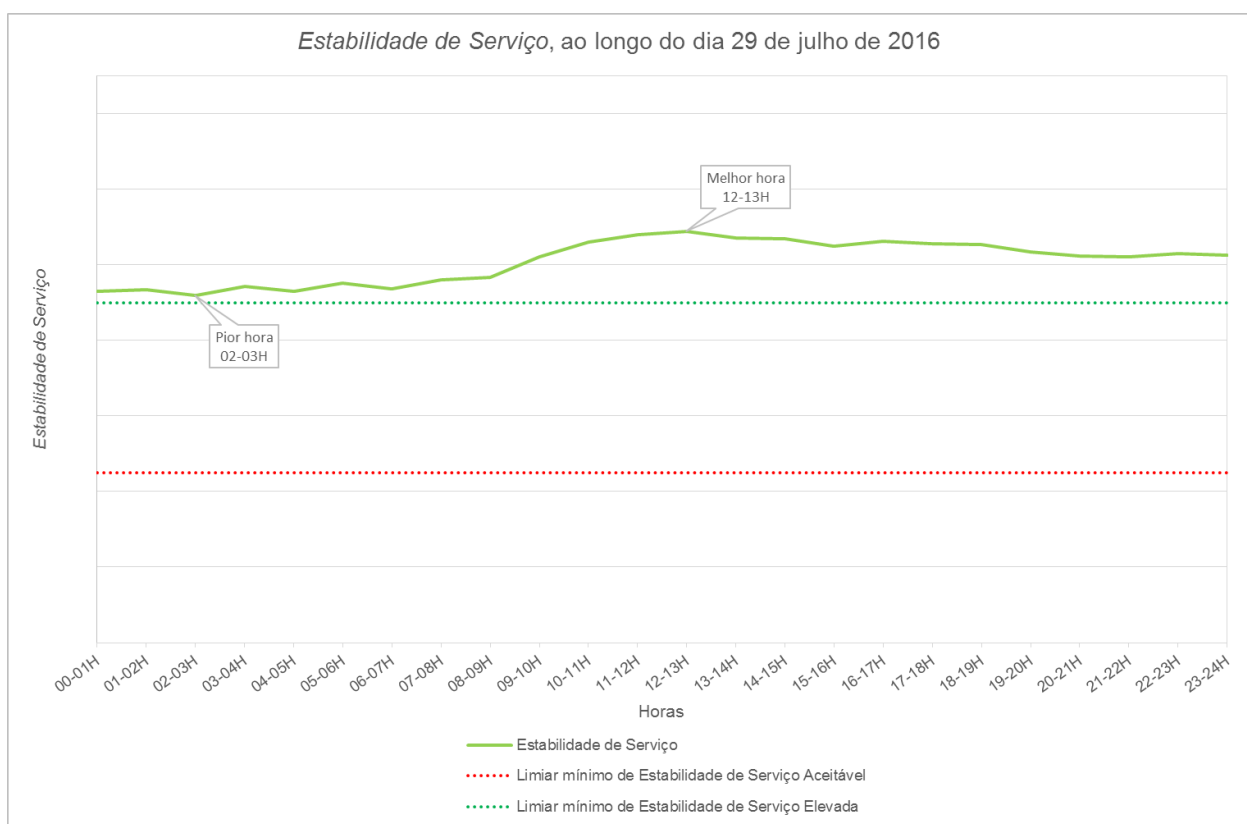
Figura 32 – Estabilidade de Serviço, ao longo do pior dia de julho de 2016
