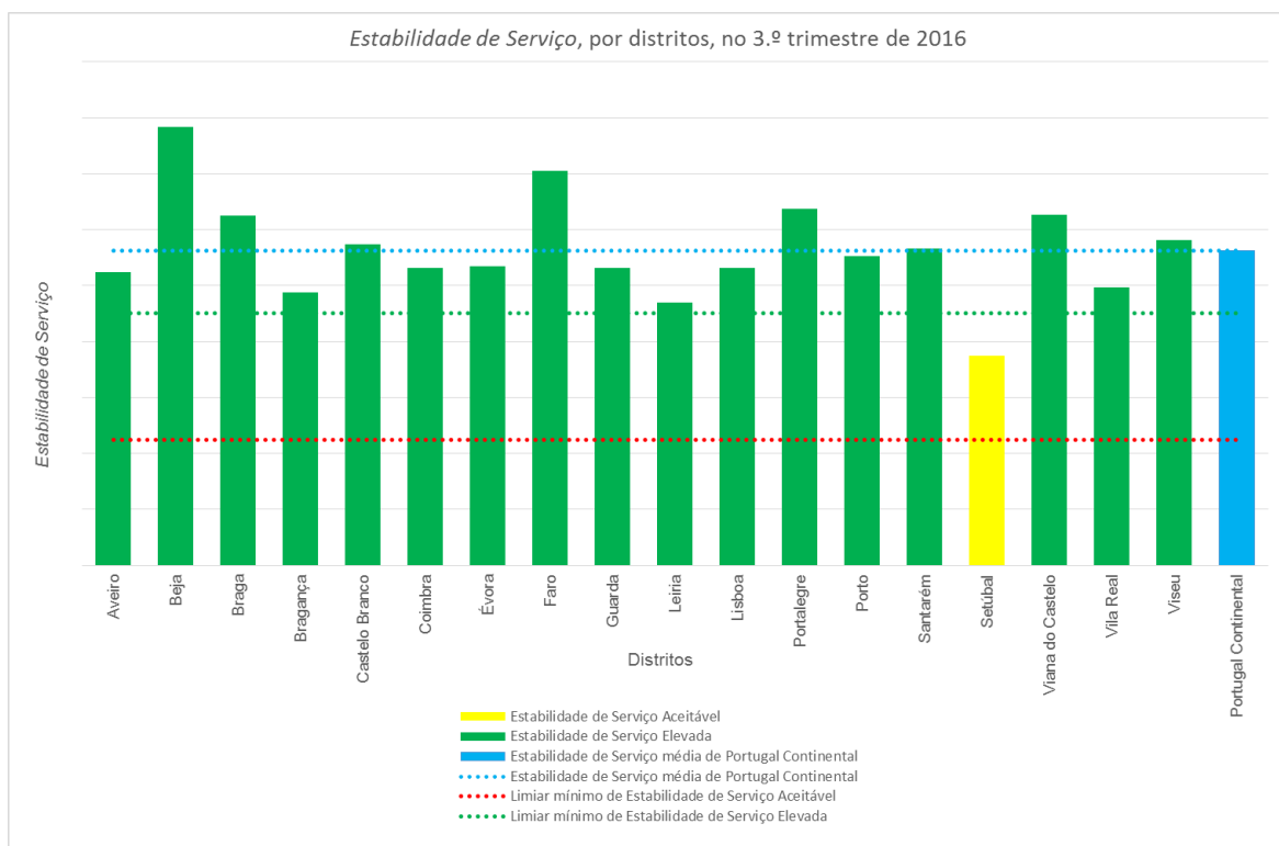
Figura 43 – Gráfico da Estabilidade de Serviço, por distritos, no 3.º trimestre de 2016
