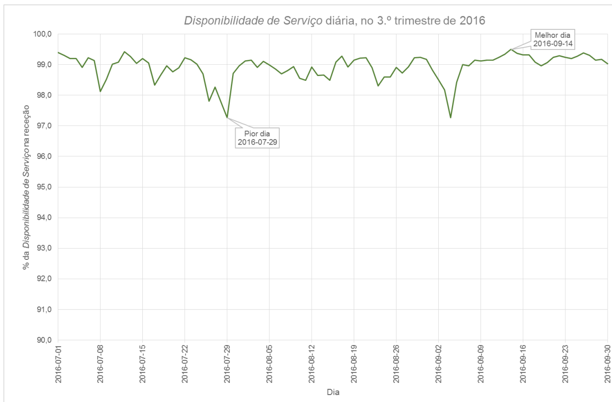
Figura 6 – Disponibilidade de Serviço em cada dia, no 3.º Trimestre de 2016
