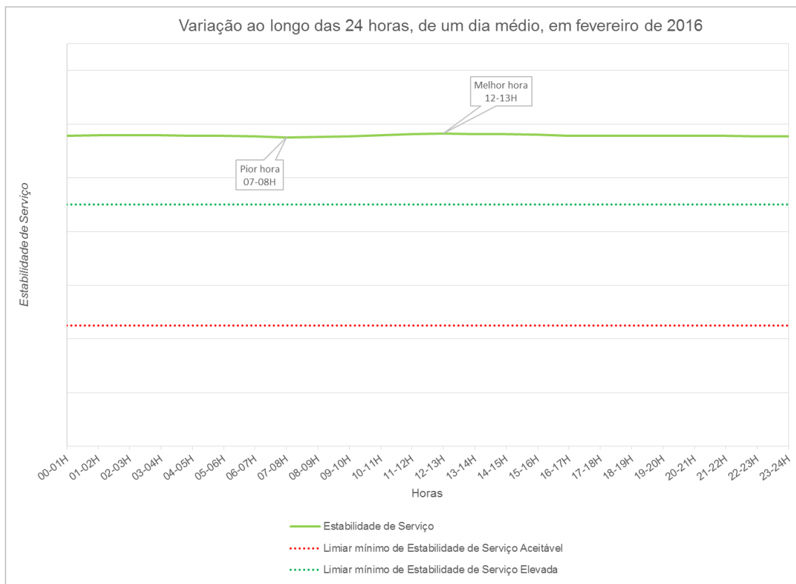
Figura 37 – Estabilidade de Serviço, nas 24 horas de um dia médio, do mês de fevereiro de 2016
