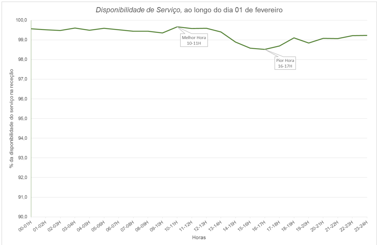
Figura 14 – Disponibilidade de Serviço, ao longo do pior dia de fevereiro de 2016
