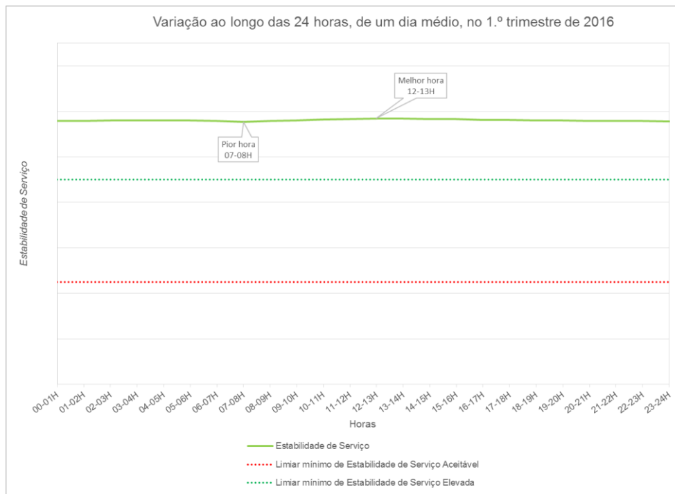
Figura 35 – Estabilidade de Serviço, nas 24 horas de um dia médio, do 1.º trimestre de 2016
