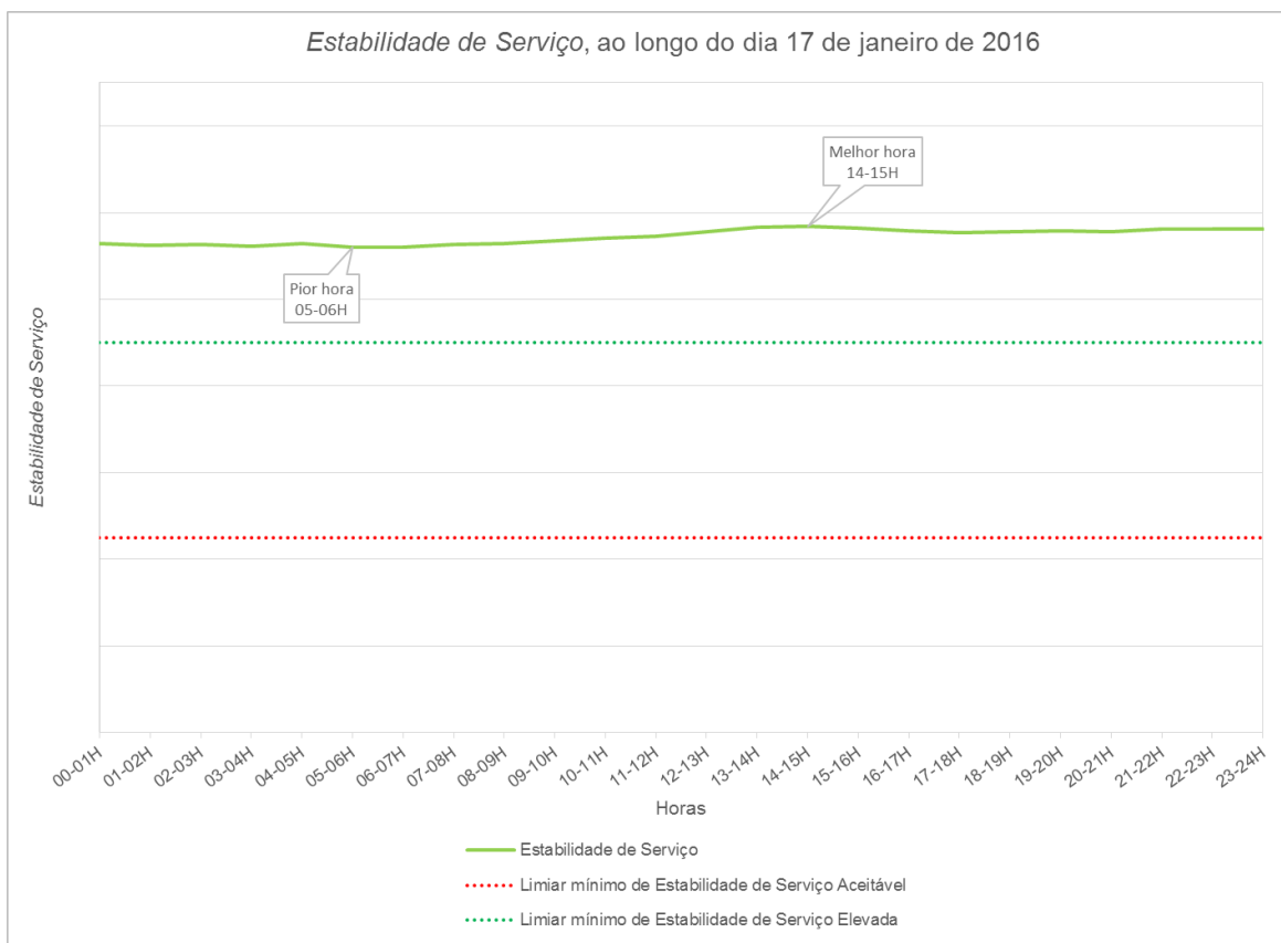
Figura 32 – Estabilidade de Serviço, ao longo do pior dia de janeiro de 2016
