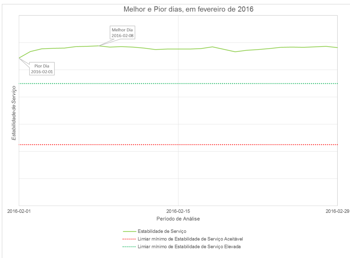
Figura 52 – Estabilidade de Serviço em cada dia, no mês de fevereiro de 2016
