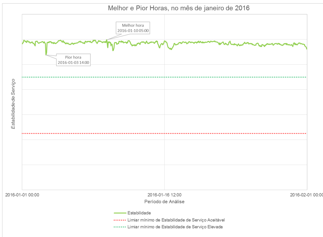
Figura 40 – Estabilidade de Serviço, hora a hora, ao longo do mês de janeiro de 2016
