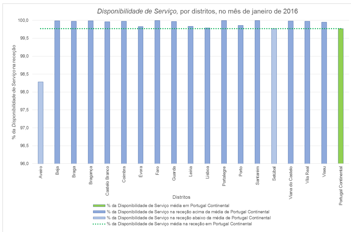
Figura 18 – Gráfico da Disponibilidade de Serviço, por distritos, no mês de janeiro de 2016
