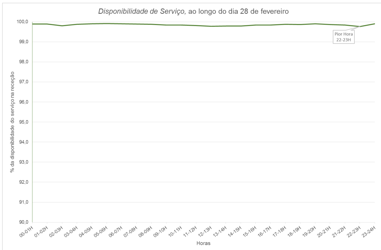
Figura 11 – Disponibilidade de Serviço, ao longo do melhor dia de fevereiro de 2016
