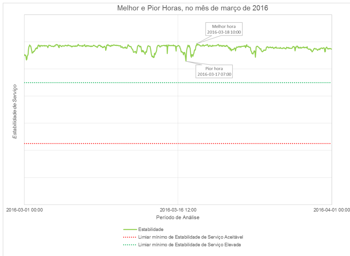
Figura 42 – Estabilidade de Serviço, hora a hora, ao longo do mês de março de 2016
