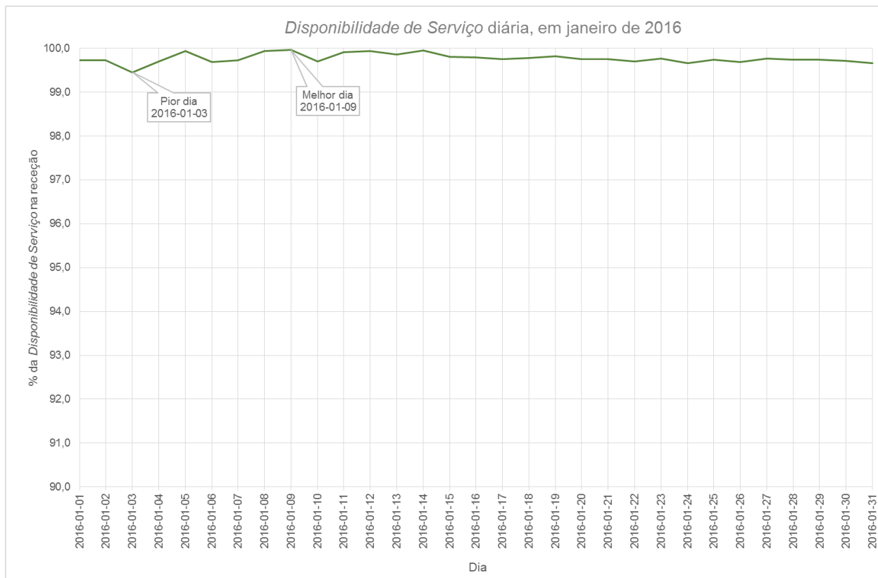
Figura 7 – Disponibilidade de Serviço em cada dia, no mês de janeiro de 2016
