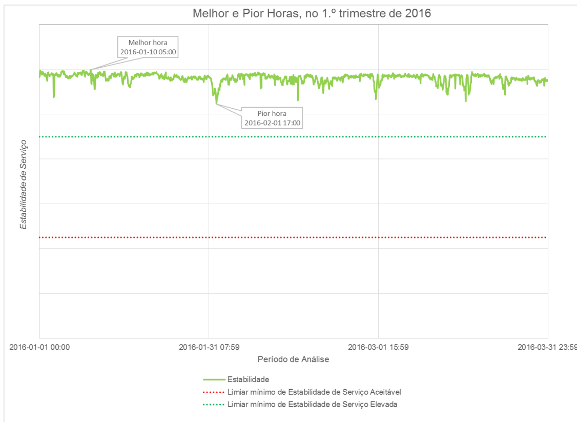
Figura 39 – Estabilidade de Serviço, hora a hora, ao longo do 1.º trimestre de 2016
