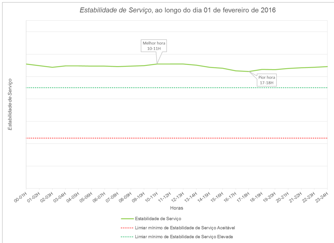
Figura 33 – Estabilidade de Serviço, ao longo do pior dia de fevereiro de 2016
