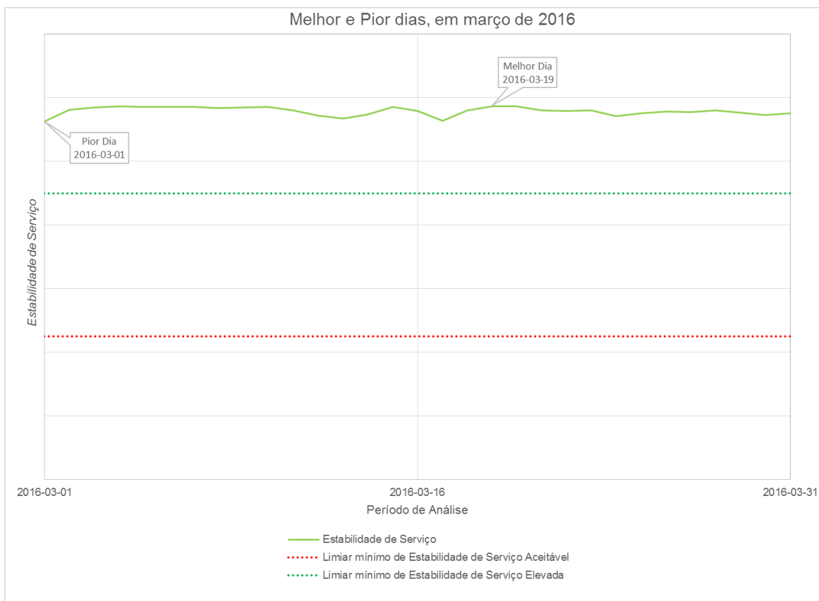
Figura 28 – Estabilidade de Serviço, em cada dia, do mês de março de 2016
