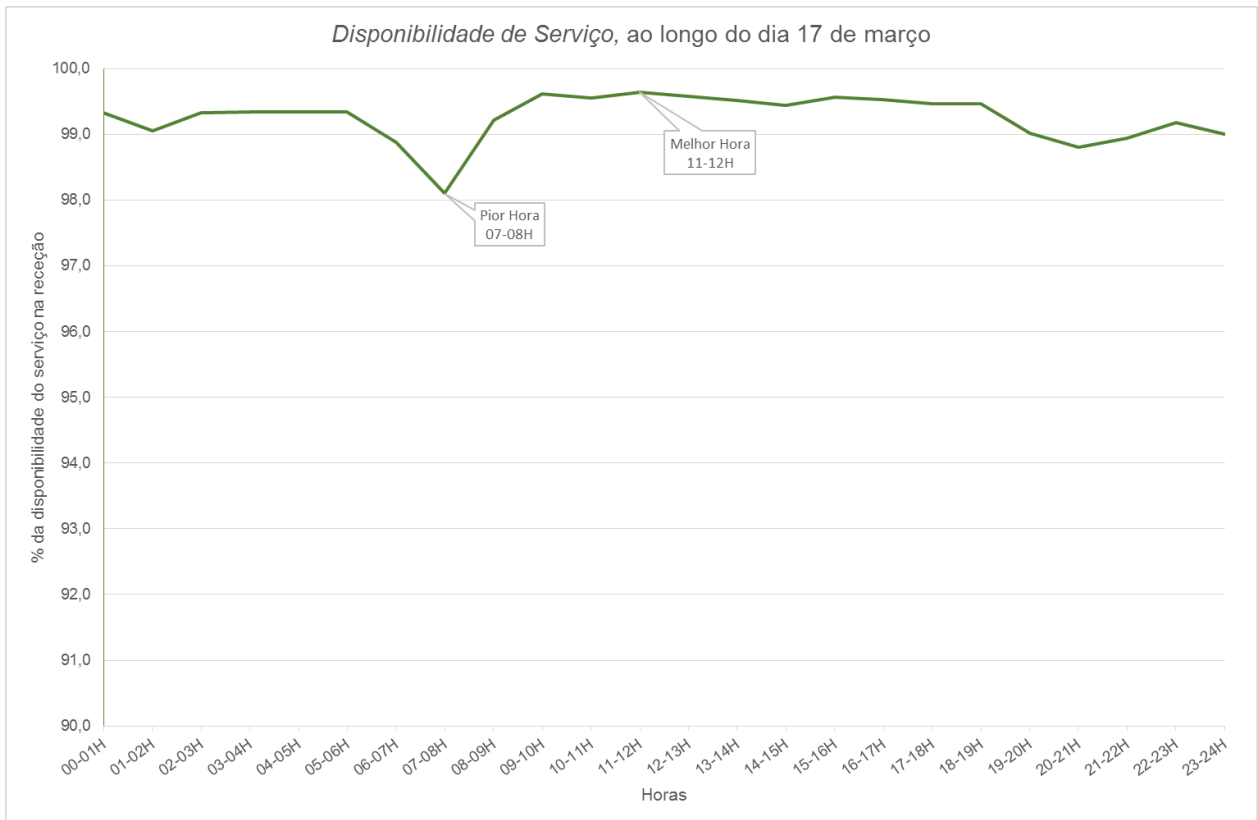
Figura 15 – Disponibilidade de Serviço, ao longo do pior dia de março de 2016
